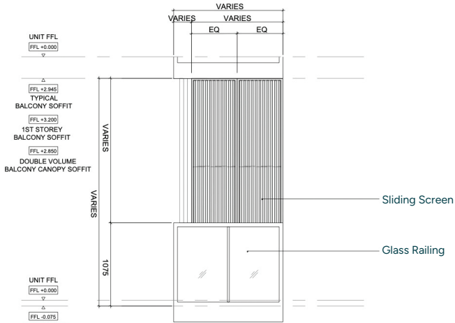
阳台立面图1 (全封闭)
